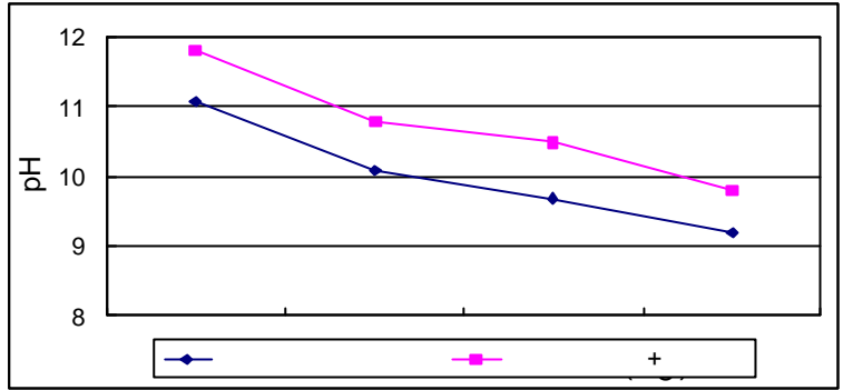
그림 6. 수증불분리혼화제 첨가량과 pH와의 관계
