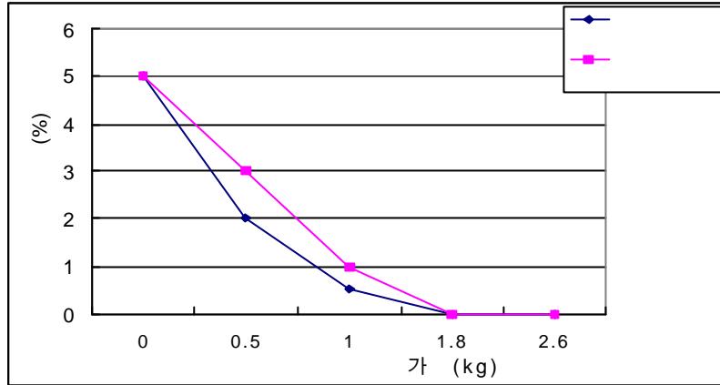
그림 2. 수중불분리혼화제의 첨가량과 블리딩율의 관계
