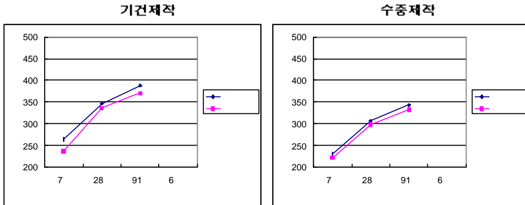
그림 9. 수중불분리혼화제 + 방청제의 압축강도 결과
