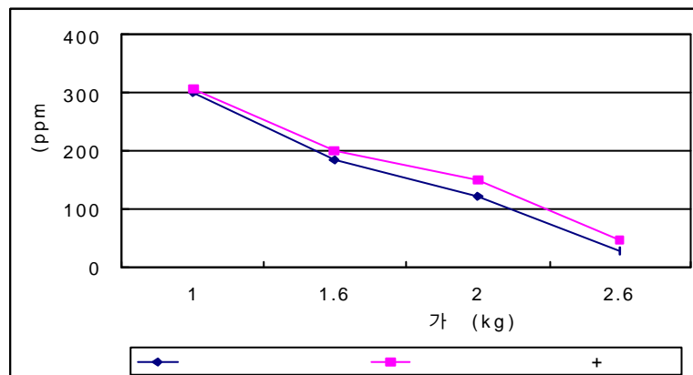
그림 5. 수중불분리혼화제 첨가량과 탁도와의 관계
