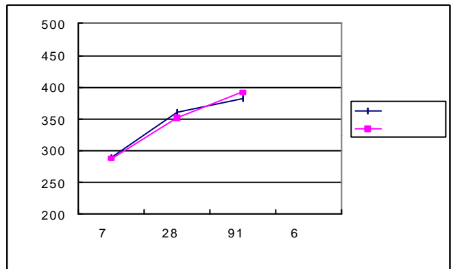
그림 7. 일반콘크리트 + 방침제(액상)의 압축강도 결과
