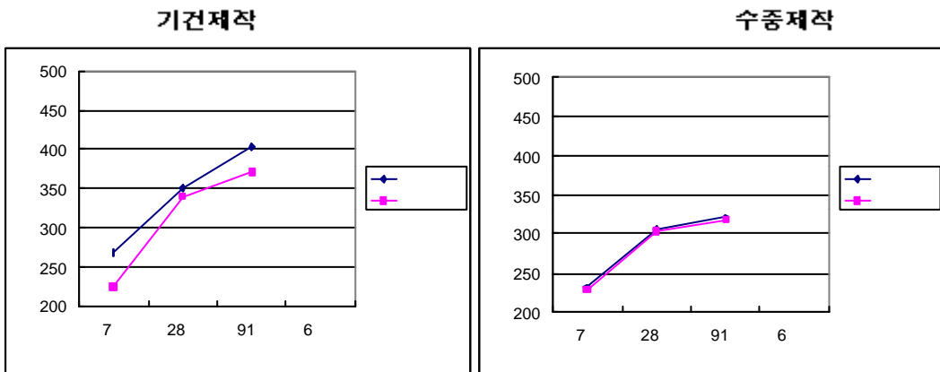
그림 8. 수증불분리혼화제의 압축강도 결과
