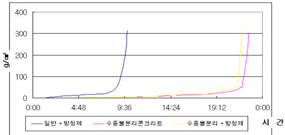
그림 3. 일반+방청제, 수중불분리혼화제, 수중불분리+방청제의 응결시간 측정결과
