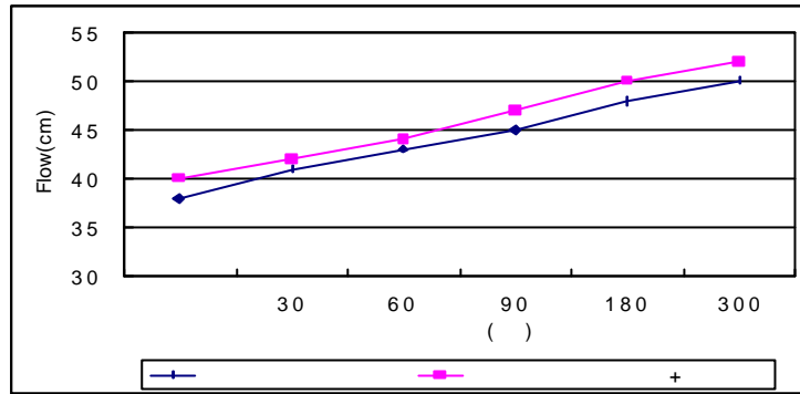
그림 4. 수중불분리혼화제와 수중불분리+방청제의 flow 경시변화 측정결과
