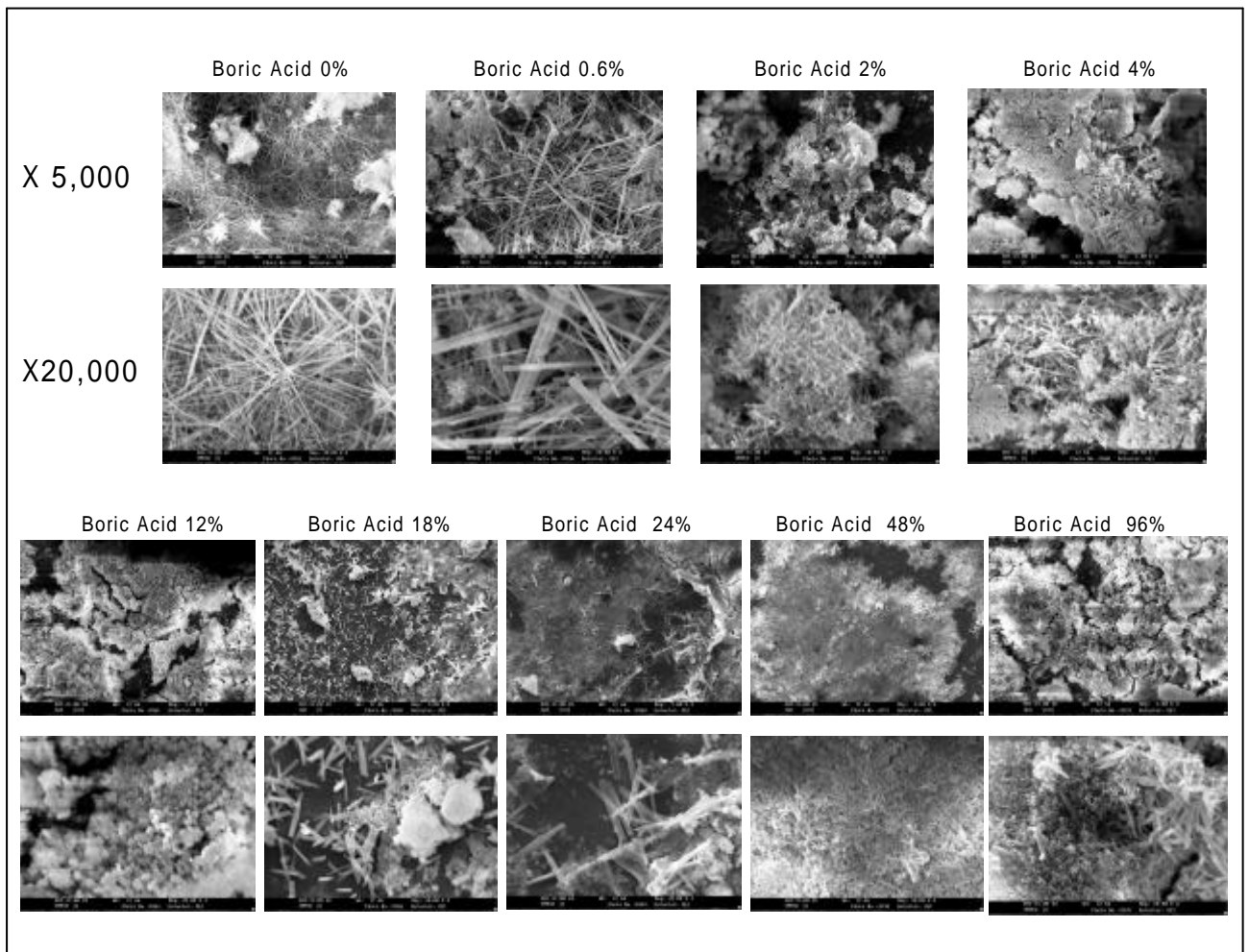
Fig. 4 SEM of synthetic ettringite with H 3 BO 3
