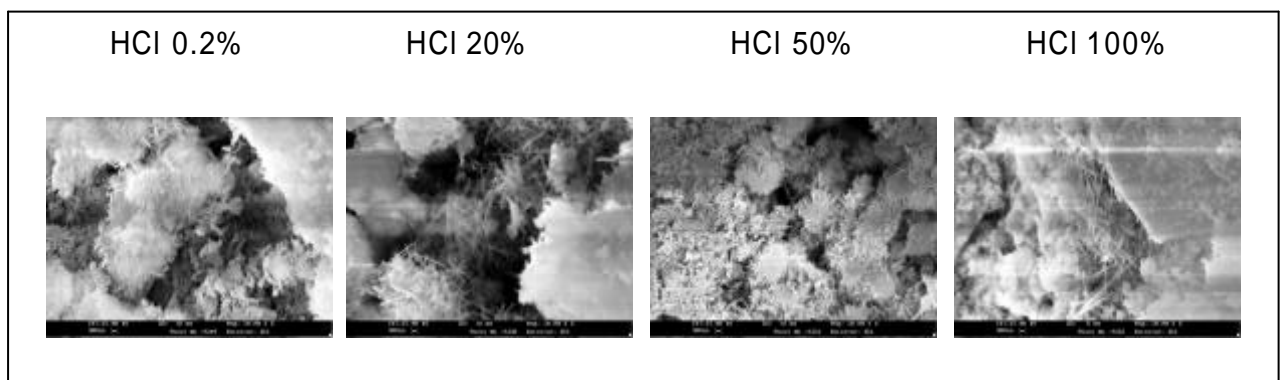
Fig. 5 SEM of synthetic ettringite with HCl
