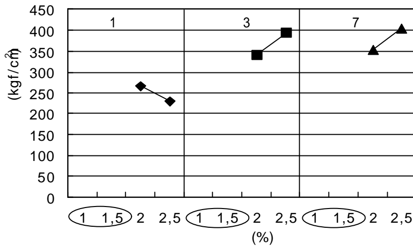
그림 11. MC 대체율에 따른 압축강도
