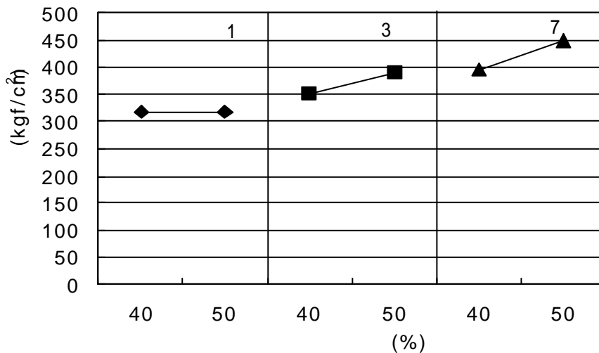
그림 13. 실리카 비율에 따른 압축강도
