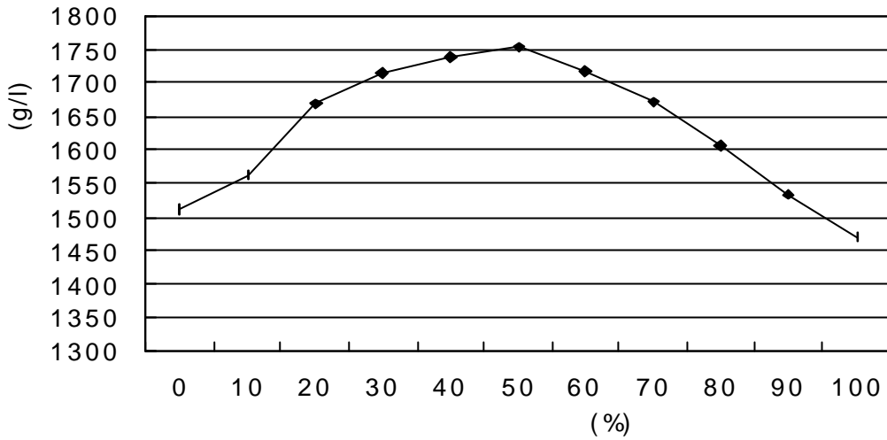
그림 12. 실리카 비율에 따른 단위용적중량
