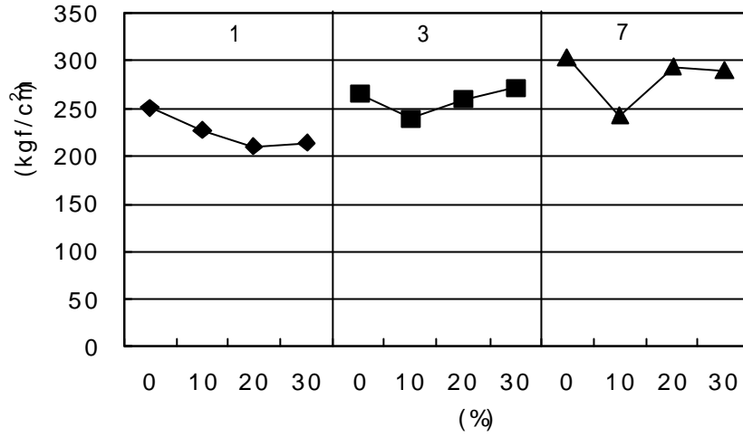
그림 7. 고로슬래그 대체율에 따른 압축강도
