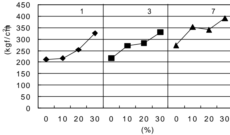
그림 9. 시멘트 혼합재(3) 대체율에 따른 압축강도
