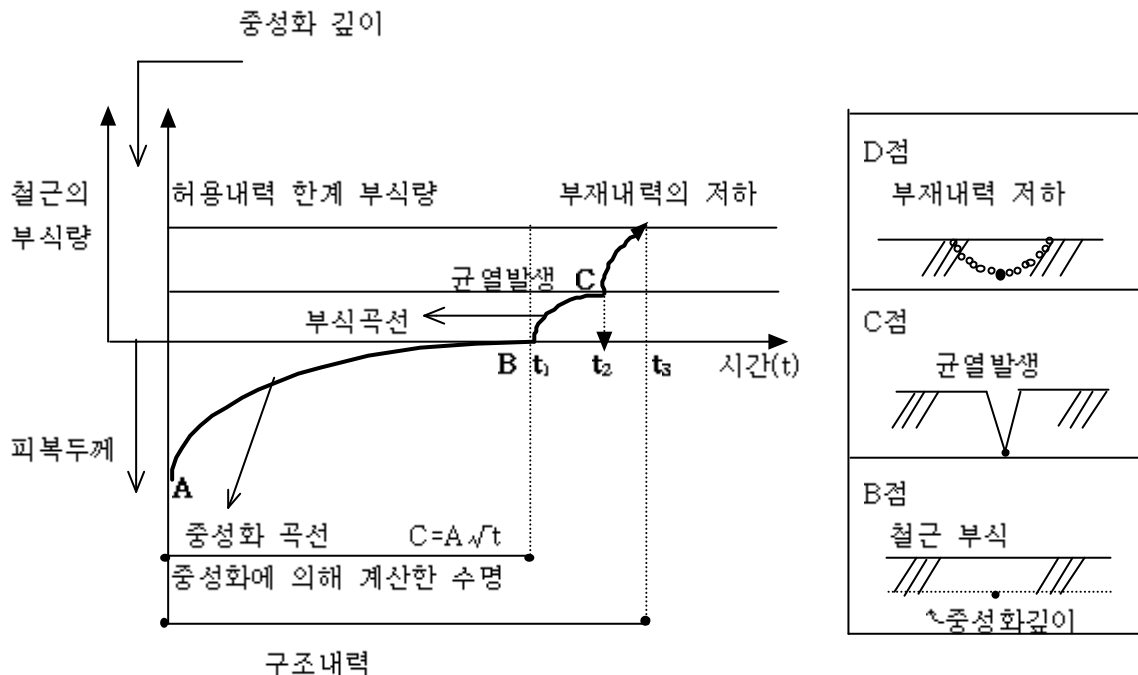
그림 1. 콘크리트 중성화와 철근부식에 의한 RC 구조물의 내용연구의 개념
