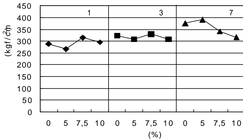
그림 10. 시멘트 혼합재(2) 대체율에 따른 압축강도
