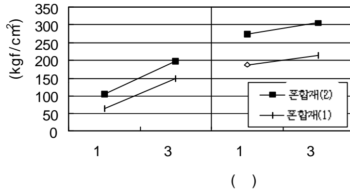
그림 6. 양생조건별 시멘트 혼화재 종류에 따른 재령별 압축강도
