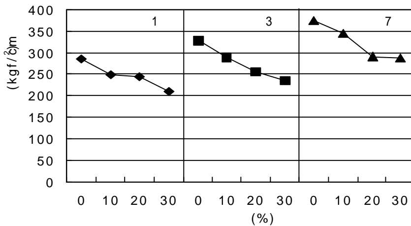
그림 8. 플라이 애쉬 대체율에 따른 압축강도
