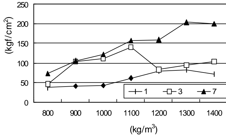
그림 5. 분체량에 따른 재령별 압축강도
