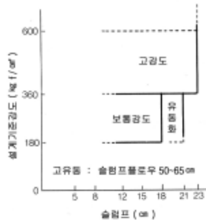
<그림-5> 일본건축학회 표준시방서에 따른 유동성과 설계기준강도의 관계 5)
