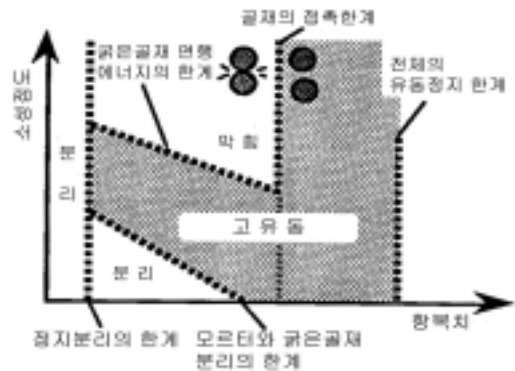
<그림-3> 간극통과성에 미치는 모르터의 레올로지 특성의 영향 3)
