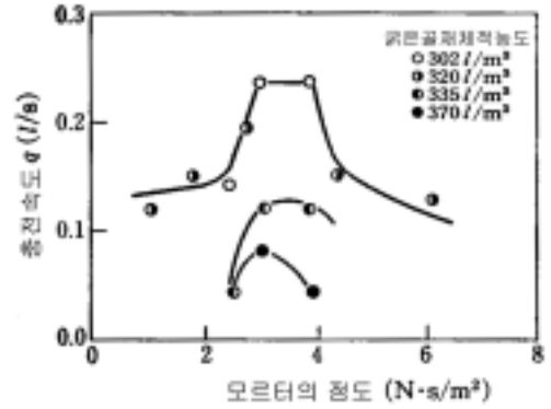
<그림-2> 모르터의 점도와 충전성의 관계 2)
