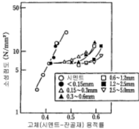
<그림-4> 고체용적율과 소성점도의 관계에 미치는 입자경의 영향 4)
