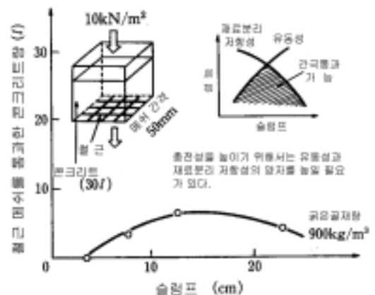
<그림-1> 슬럼프와 충전성의 관계 1)
