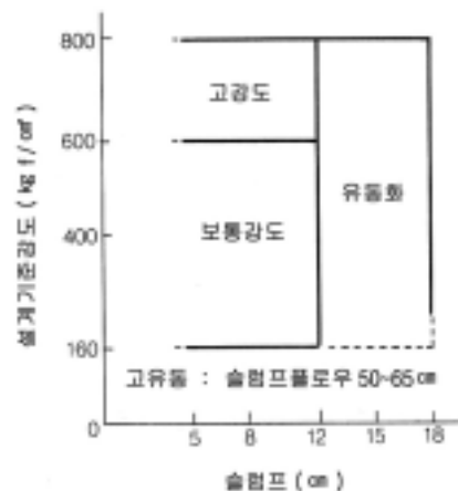
<그림-6> 일본토목학회 표준시방서에 따른 유동성과 설계기준강도의 관계 5)
